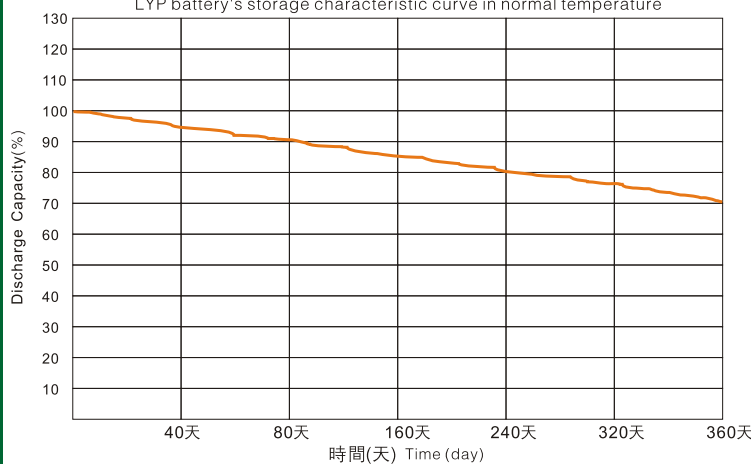
在常溫下LYP類電池的存儲特性曲線
